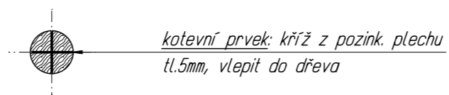
Řez - ukotvení
