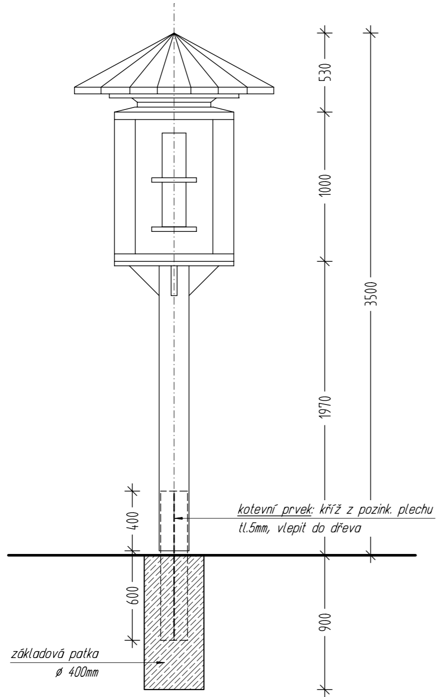
Řez - ukotvení
